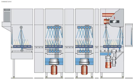
图解机器截面
